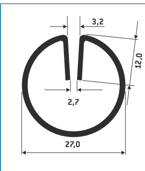
PROFILE LR 27 · 2.7
